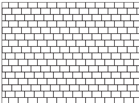
Motif G (8 x 12 Troisième appareil en long)
