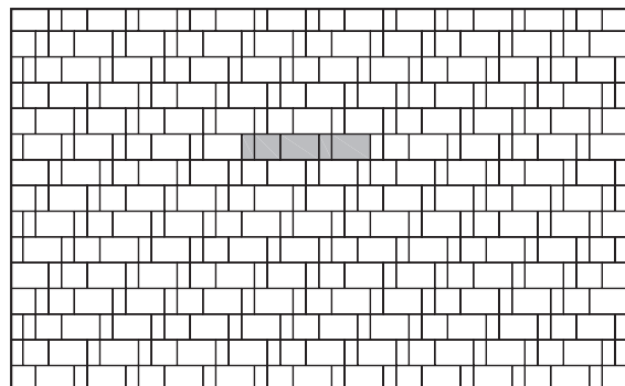
Motif D (Appareil en long emballage aléatoire)
