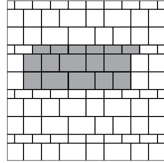
MOTIF C (Appareil en long avec emballage aléatoire)
